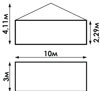
1 модуль
