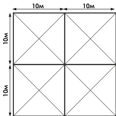
4 шатра, конф. №8
